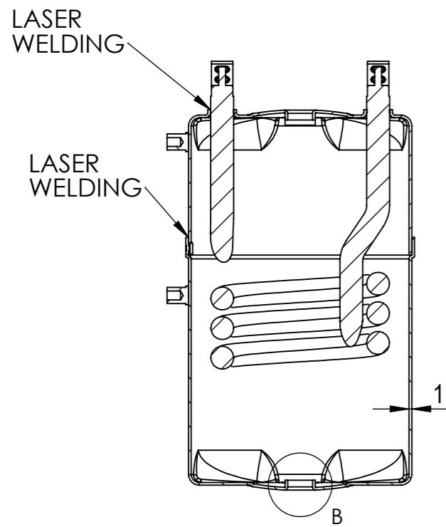
SEZIONE A-A
