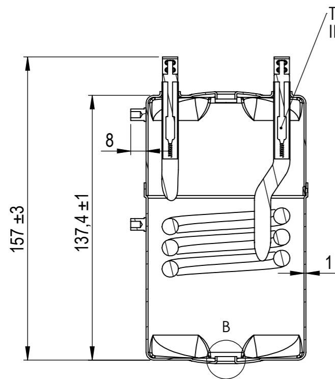
SEZIONE A-A
